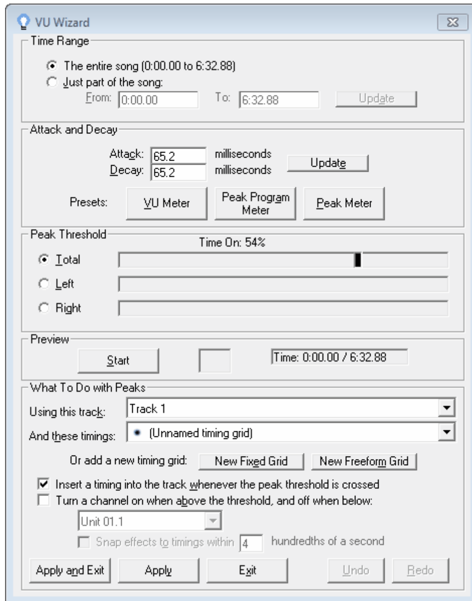
The VU Wizard
